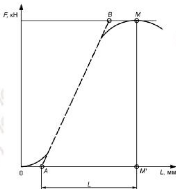
Рисунок 3 — График определения деформации
