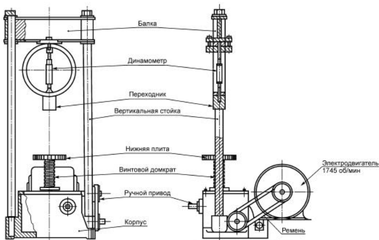
Рисунок 2 — Схема испытательной установки
